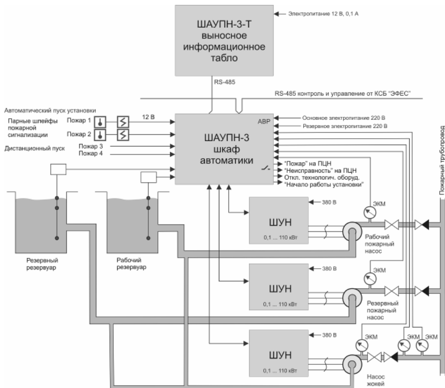
Рис. 1.1 Установка автоматическая пожаротушения. Схема общая.
